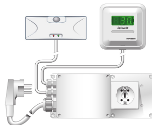
Spisvakt 230V/400V 230V 25A, Art.nr. 6490 400V 16A, Art.nr. 6491
